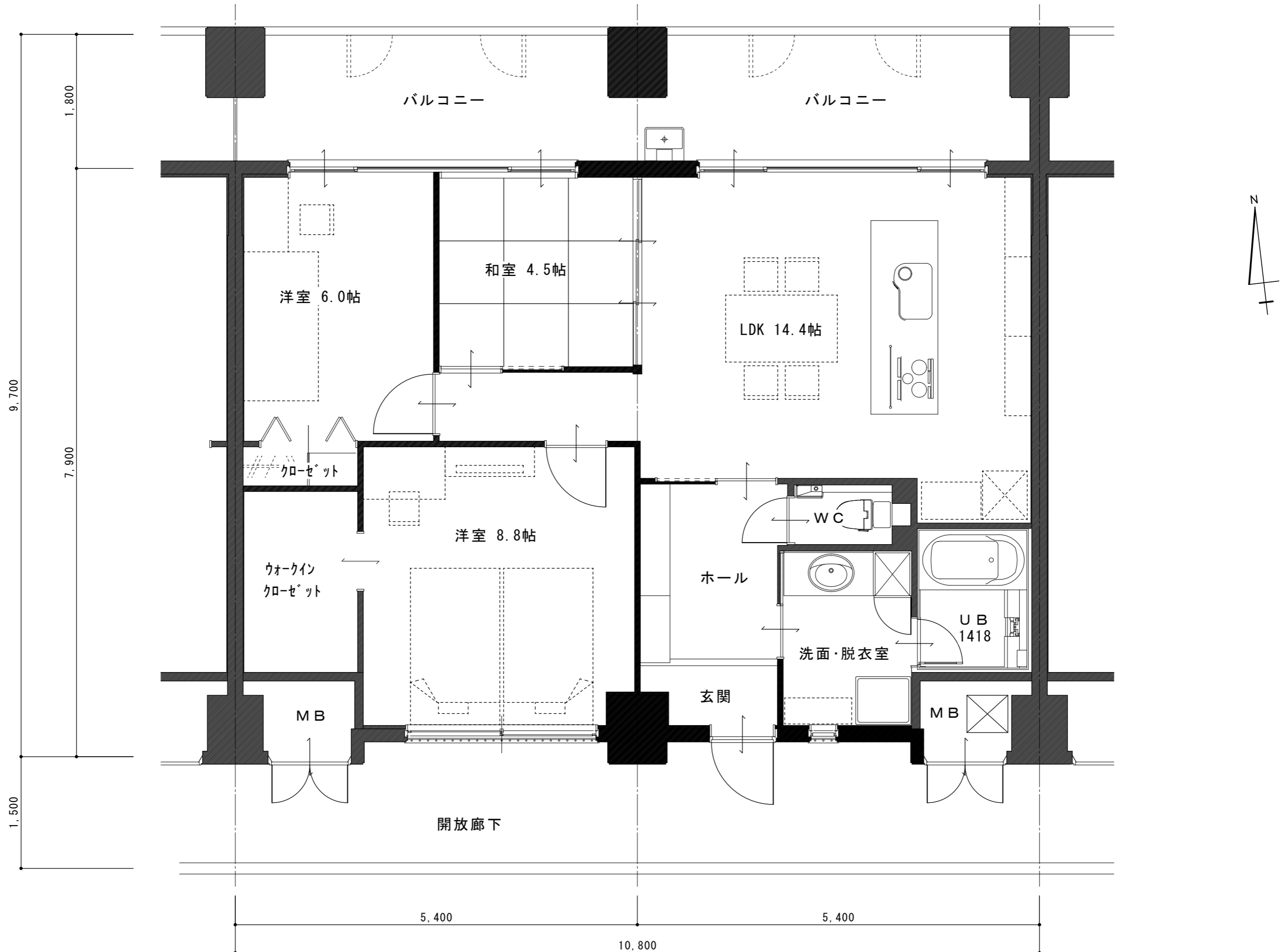
住戸Bタイプ平面図 1/50
