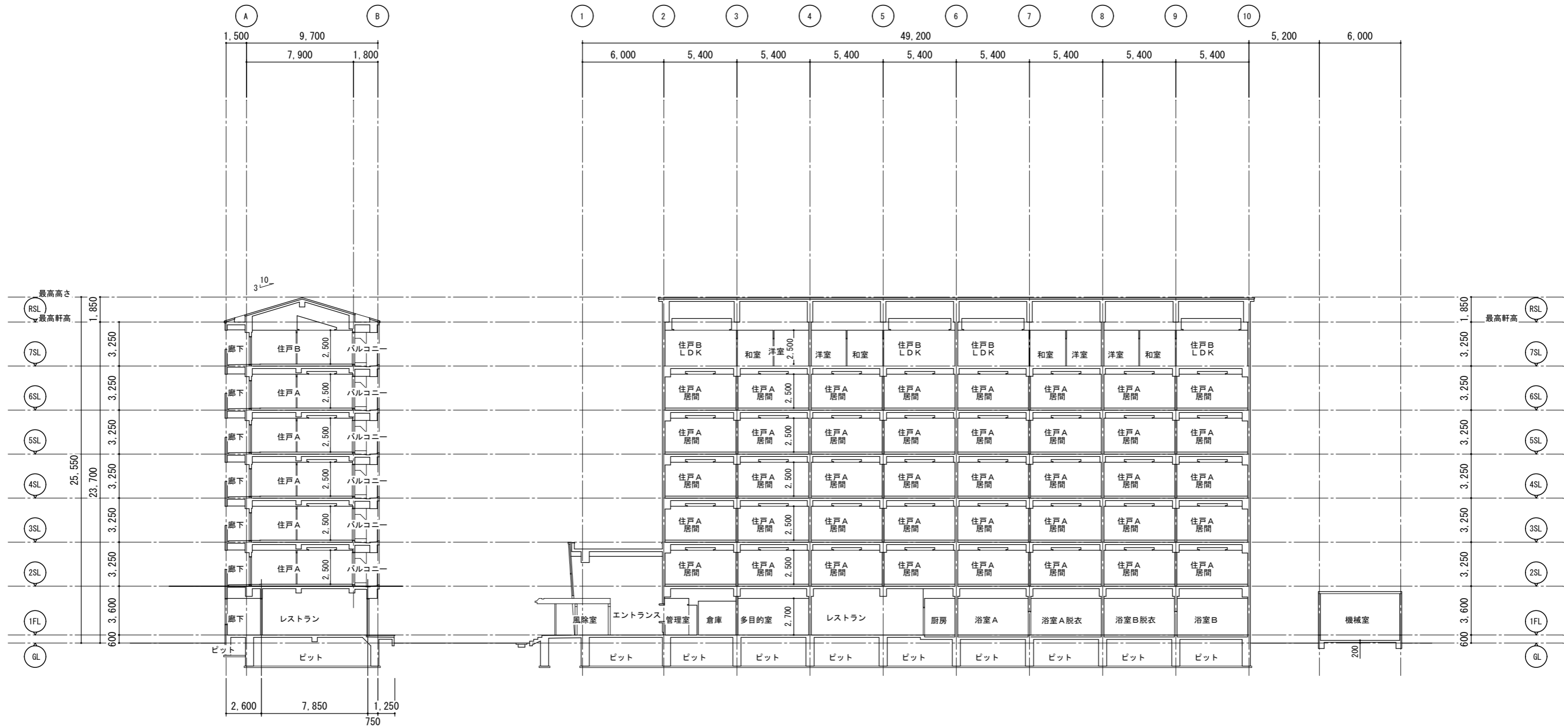
断面図
